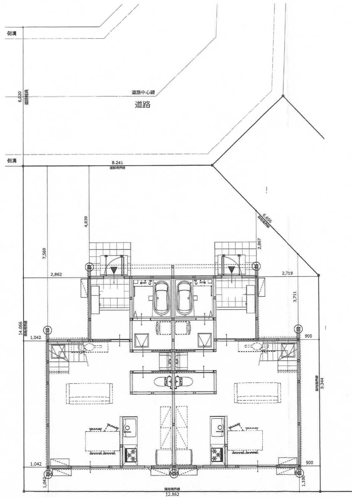
敷地配置図
