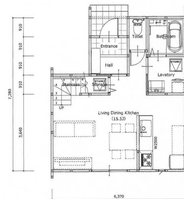
1階平面図
