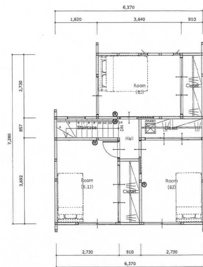
2階平面図
